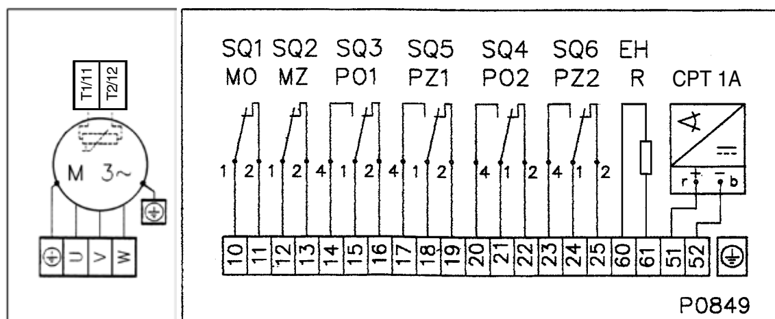
Elektromotor
