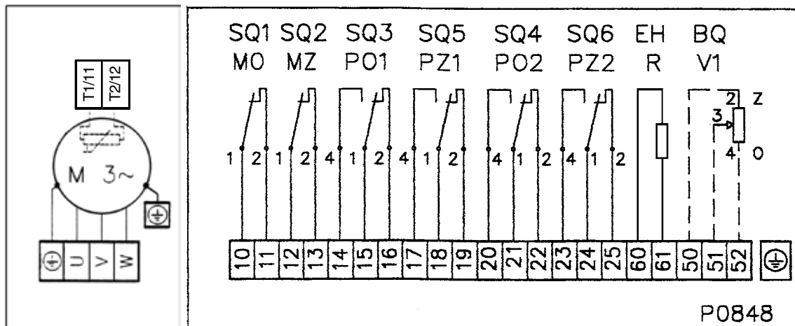
Elektromotor
